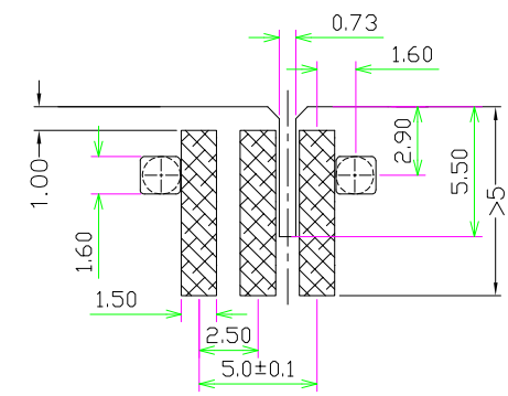
P.C.Board layout
